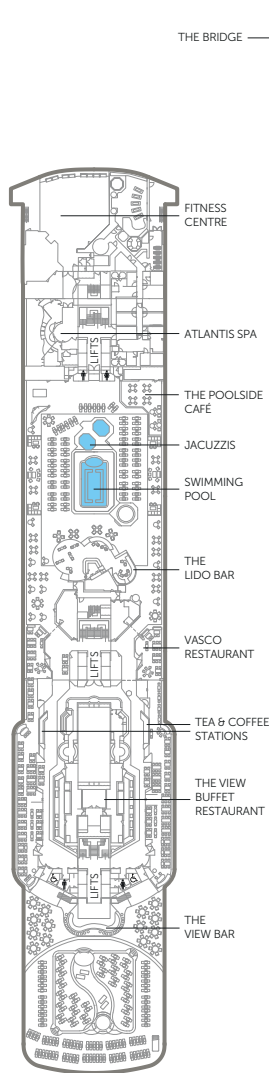
Lido Deck 8
